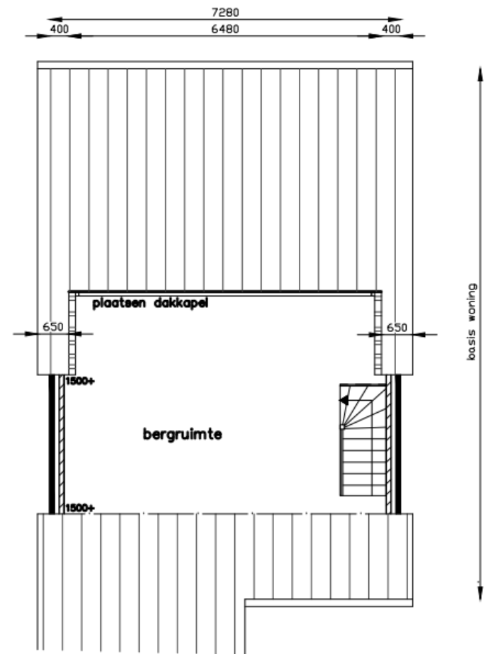
GEWIJZIGDE VERDIEPING
