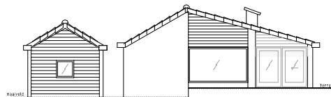
ACHTERGEVEL NIEUW
