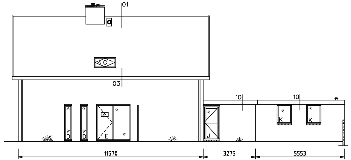
Zijgevel Rechts Bestaand
