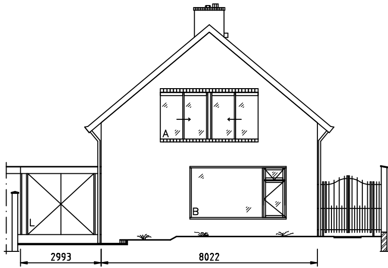
Voorgevel Bestaand
