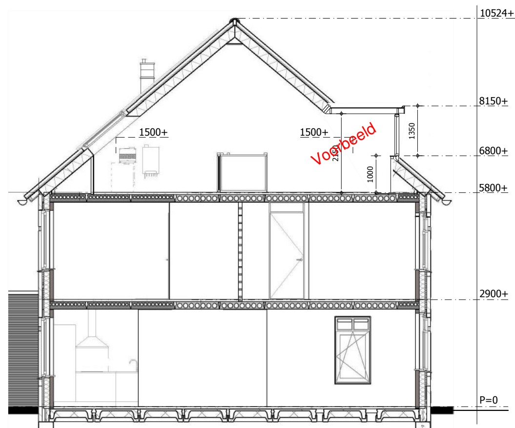
GEWIJZIGDE DOORSNEDE
