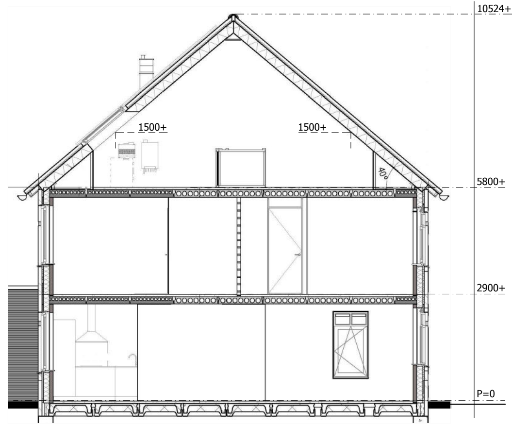
BESTAANDE DOORSNEDE
