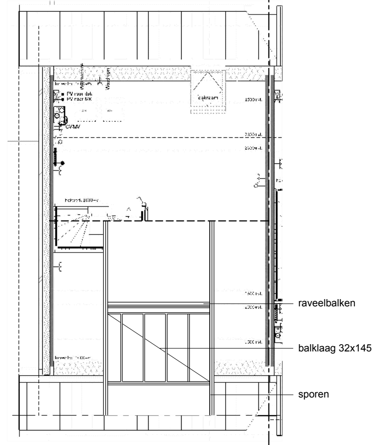
KAPPLAN
